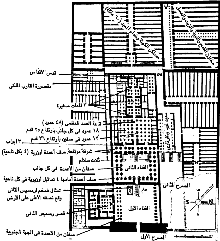
شكل ١٧٠ - رسم تخطيطي للرمسيوم وهو المعبد الجنائزى لرمسيس الثاني .
